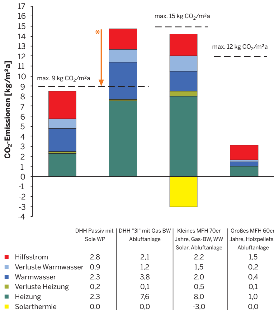
Abbildung 4-2: Beispiele aufsummierter CO 2 -Emissionen für verschiedene Gebäudetypen und Versorgungsvarianten [kg/m 2 a]
