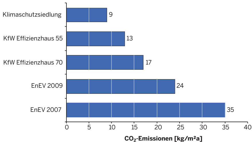
Abbildung 4-1: Vergleich der CO 2 -Emissionen für eine Doppelhaushälfte (Neubau) bei unterschiedlichen Gebäudestandards
