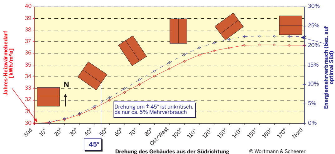
Abbildung 3-1: Jahres-Heizwärmebedarf eines aus der Südrichtung gedrehten Gebäudes mit einem Fensterflächenanteil von 70 % im Süden
